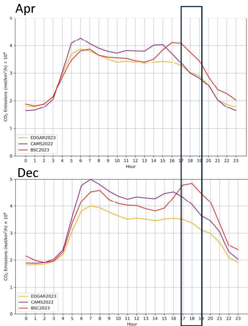
Fig Variación diurna mensual de las emisiones de CO 2 emission(mol/km²/h x10 4 ) en AMB a partir de diferentes inventarios antropogénicos en abril y diciembre.
