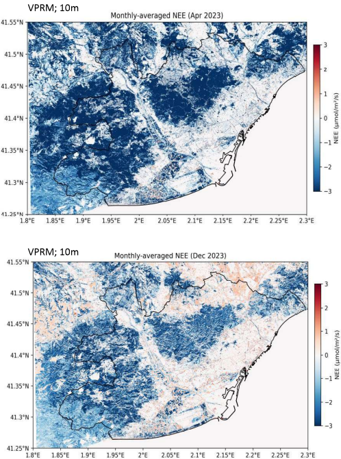
Emissiones totales mensuales (kilotoneladas C/mes) de cada clase dentro de AMB
